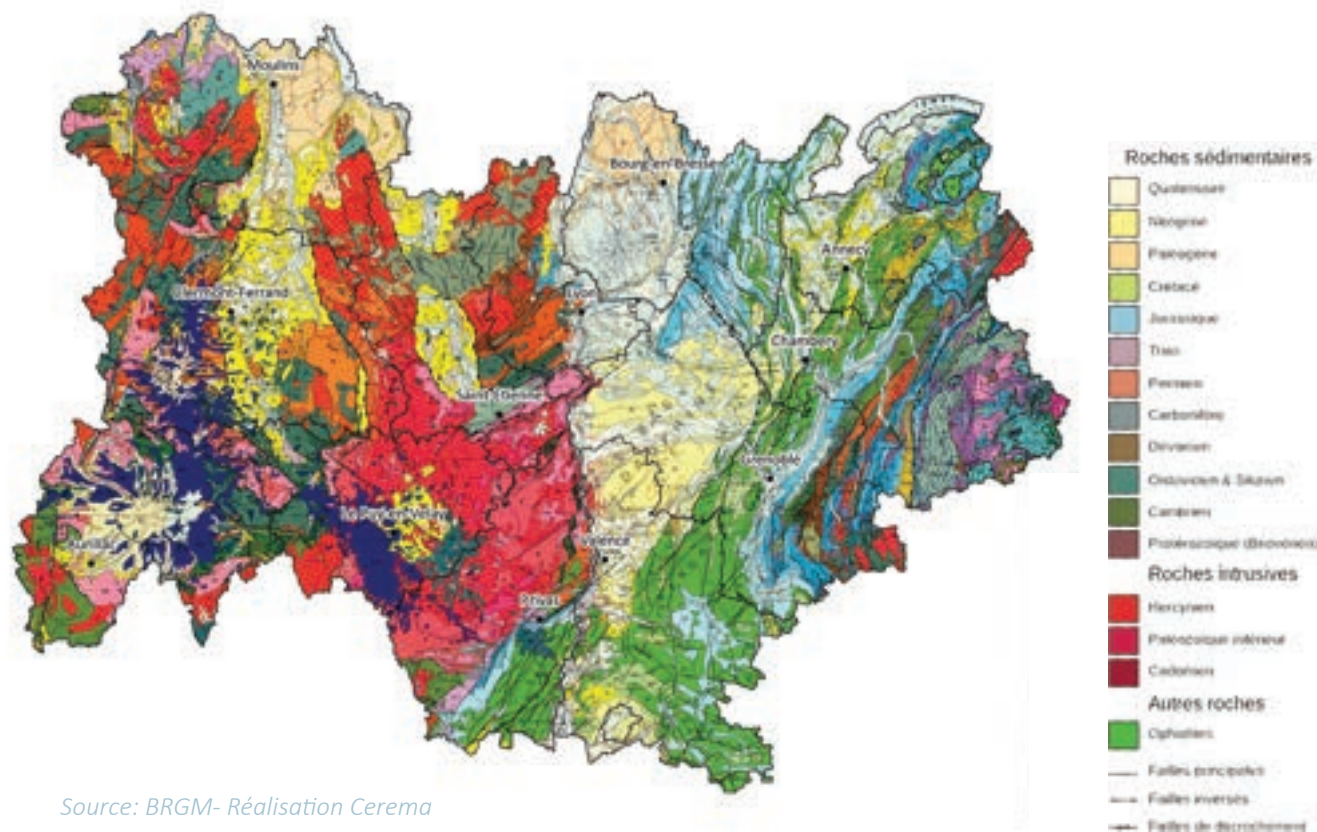
CARTE GÉOLOGIQUE
